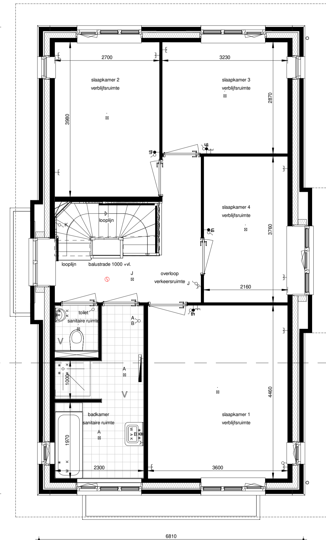
EERSTE VERDIEPING VAN SLINGELANDT V.B2 (923) Schaal 1:50
