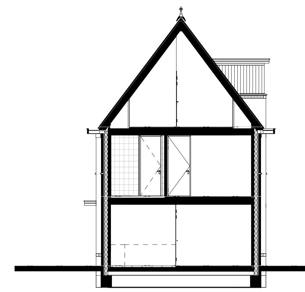
DOORSNEDE A-A Schaal 1:100
