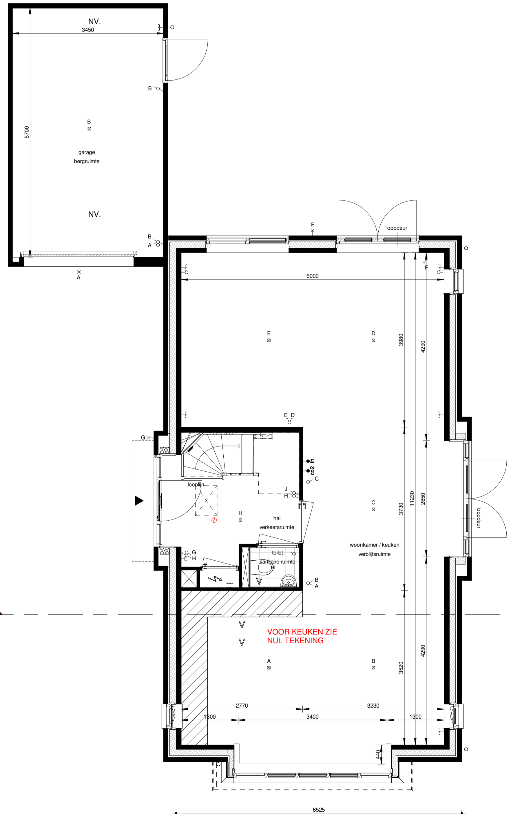
BEGANE GROND VAN SLINGELANDT V.B2 (923) Schaal 1:50
