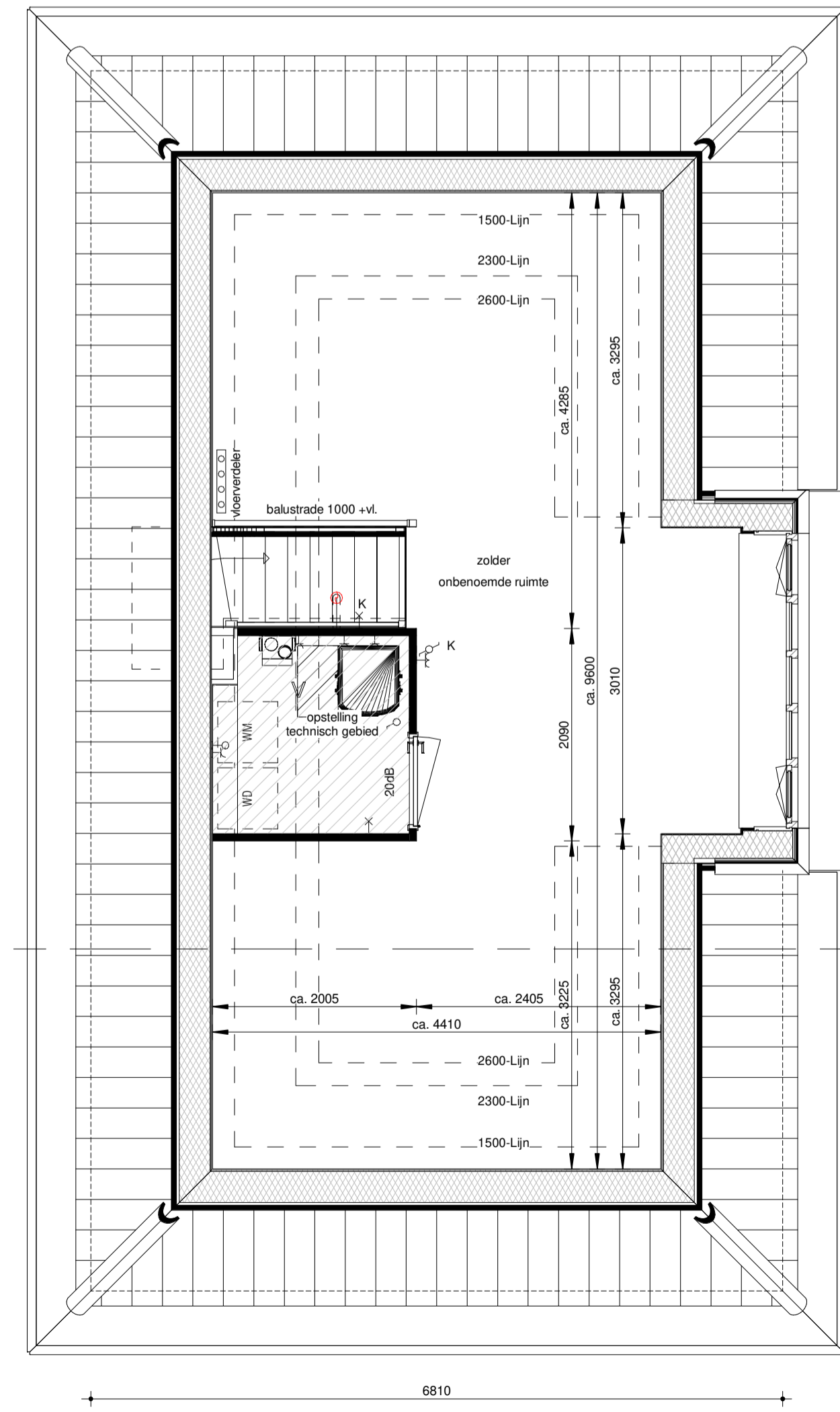
TWEDE VERDIEPING VAN SLINGELANDT V.B2 (923) Schaal 1:50
